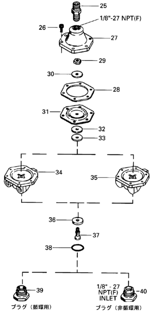
アダプター (塗料入口)
