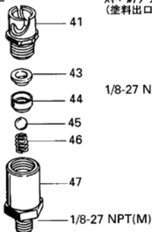
バイオネットアダプター ASSY (塗料出口) HGS-401-1
